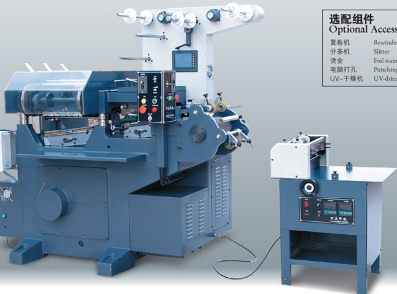
自动复卷机 Auto Rewinder
